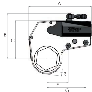
TWH430N (cuerpo de acero)
